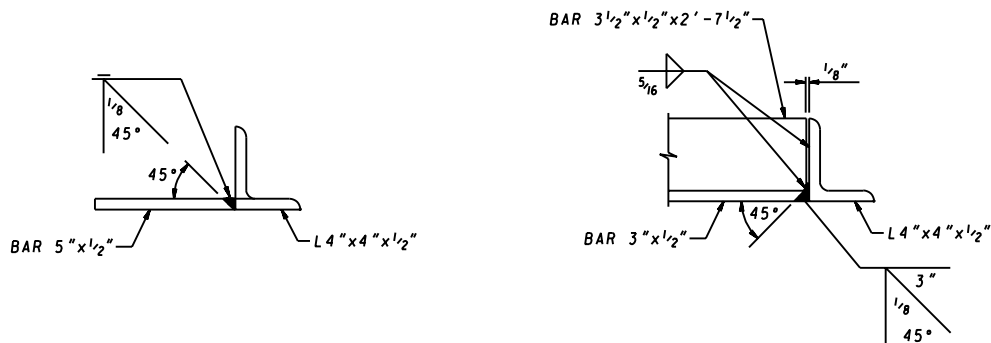
SECTION D-D
